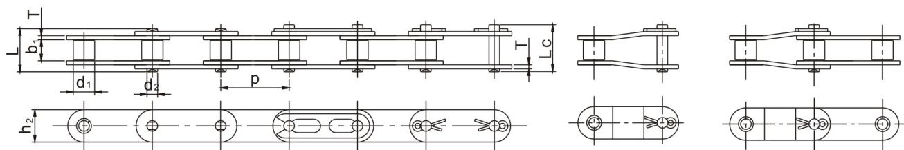
小滚子型 Small Roller Type
