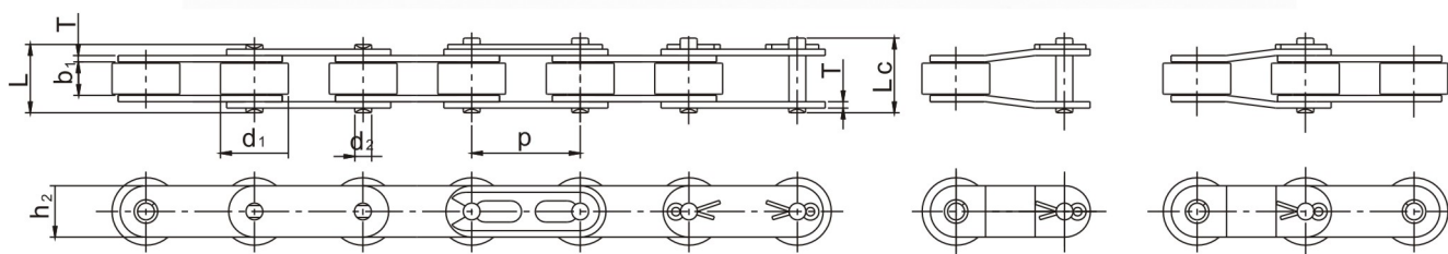
大滚子型 Large Roller Type
